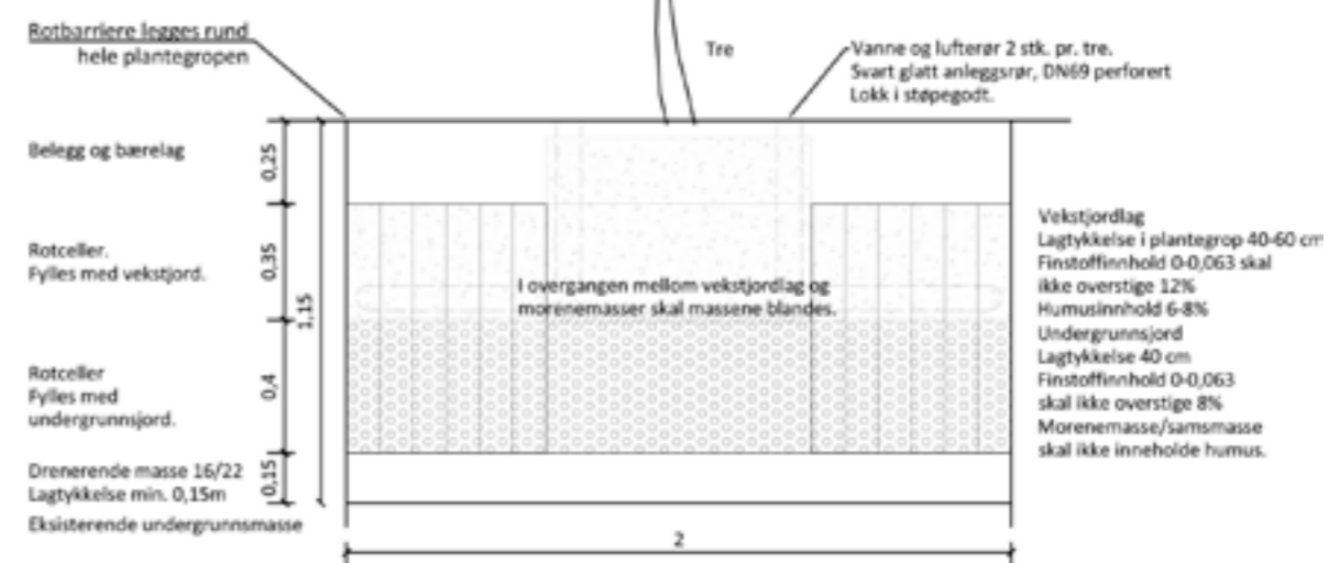
Prinsippsnitt planting av tre med armert jordoppbygning (prinsipp 4)
