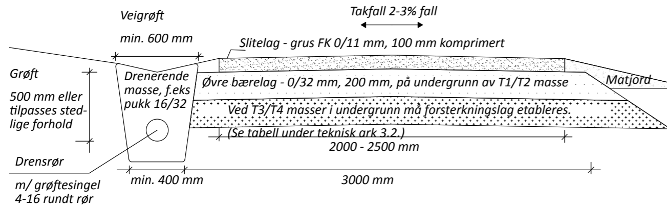
Prinsippnitt
