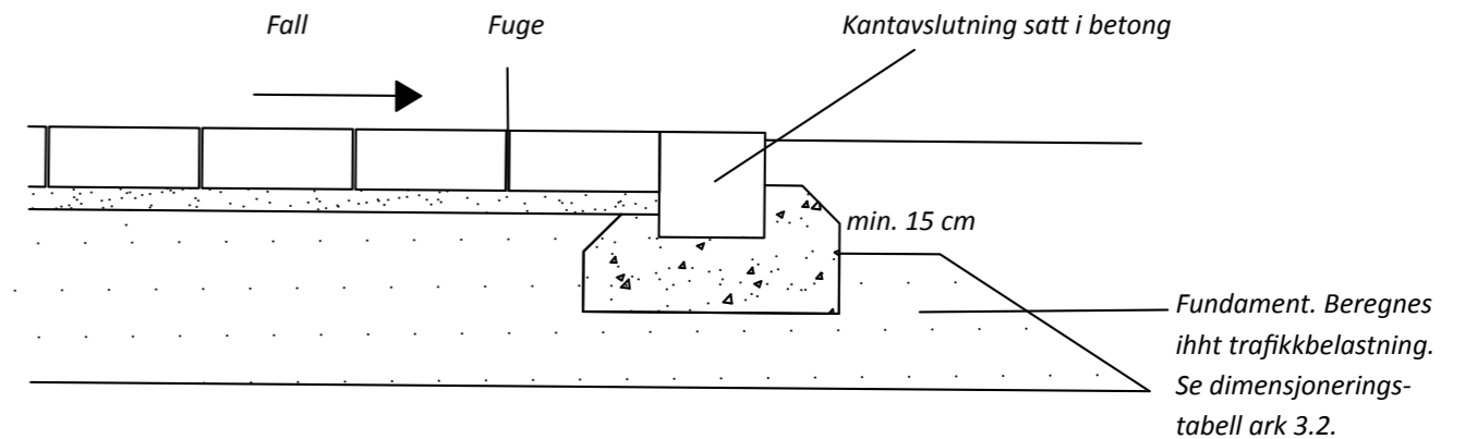
Prinsippsnitt legging av belegg med avslutning mot terreng
