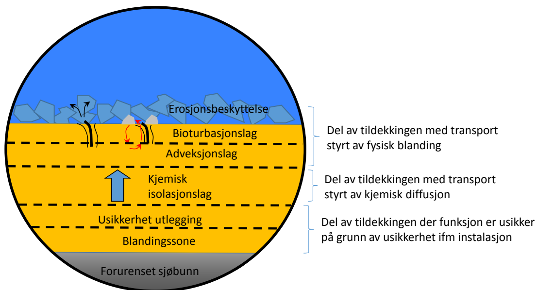
Figur 10 Tildekkingsdesign
