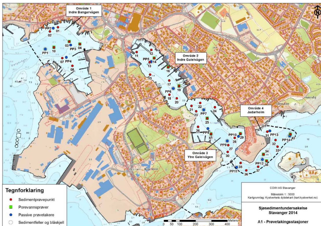
Figur 3 Inndeling i delområder fra COWI 2015
