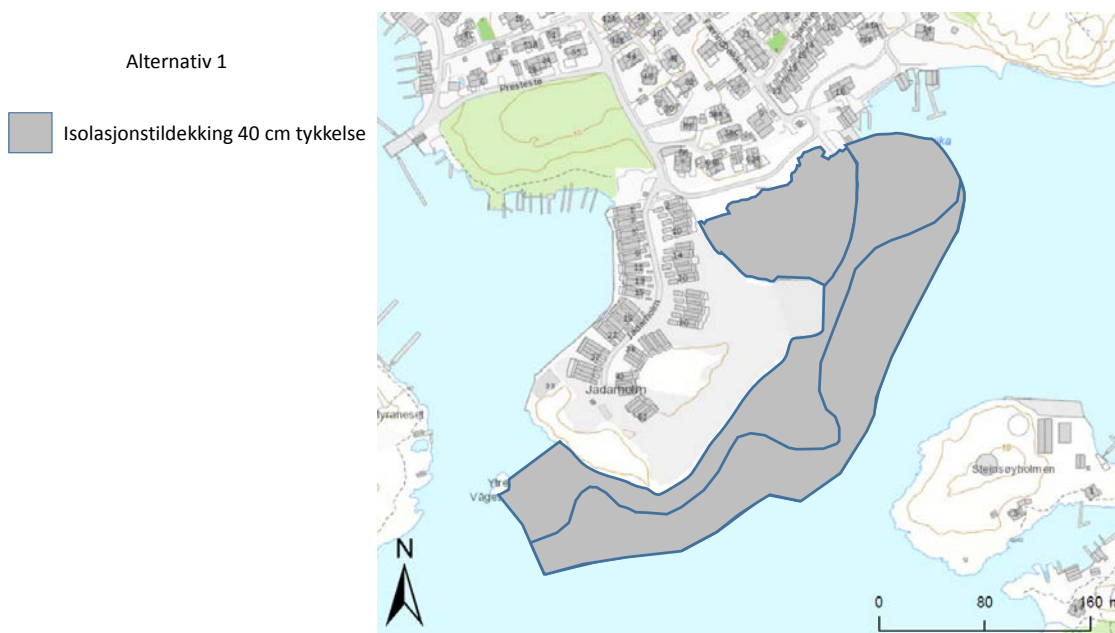
Figur 22 Arealplan for tiltaksalternativ 1 i tiltaksområde Jadarholm
