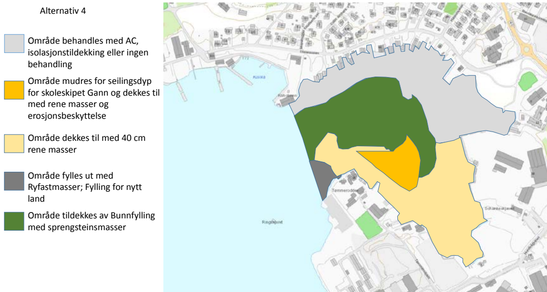
Figur 16 Planskisse Tiltaksalternativ 4 Bangarvågen
