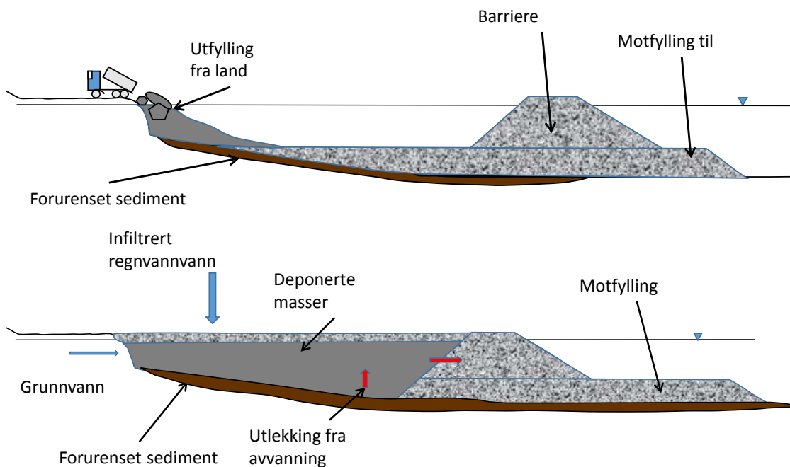
Figur 25 Skisse (ikke målsatt) av snitt gjennom strandkantdeponi. Illustrerer viktige forhold ved et slikt deponi.
