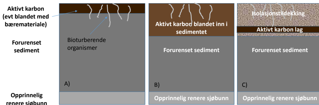
Figur 12 Illustrasjon av behandling med aktivt kull. A) Tynn tildekning sjøbunnsoverflaten. B) innblanding av AC i de øverste om lag 10 cm for å kjemisk stabilisere Hg og dioksiner i disse. C) aktivt kull som et lag i en isolasjonstildekning.
