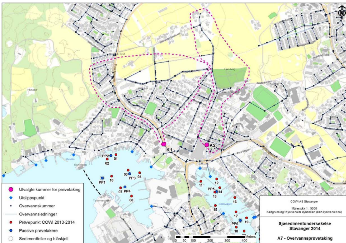
Figur 4 Overvannsnett i tiltaksområdet. Fra COWI (2015)
