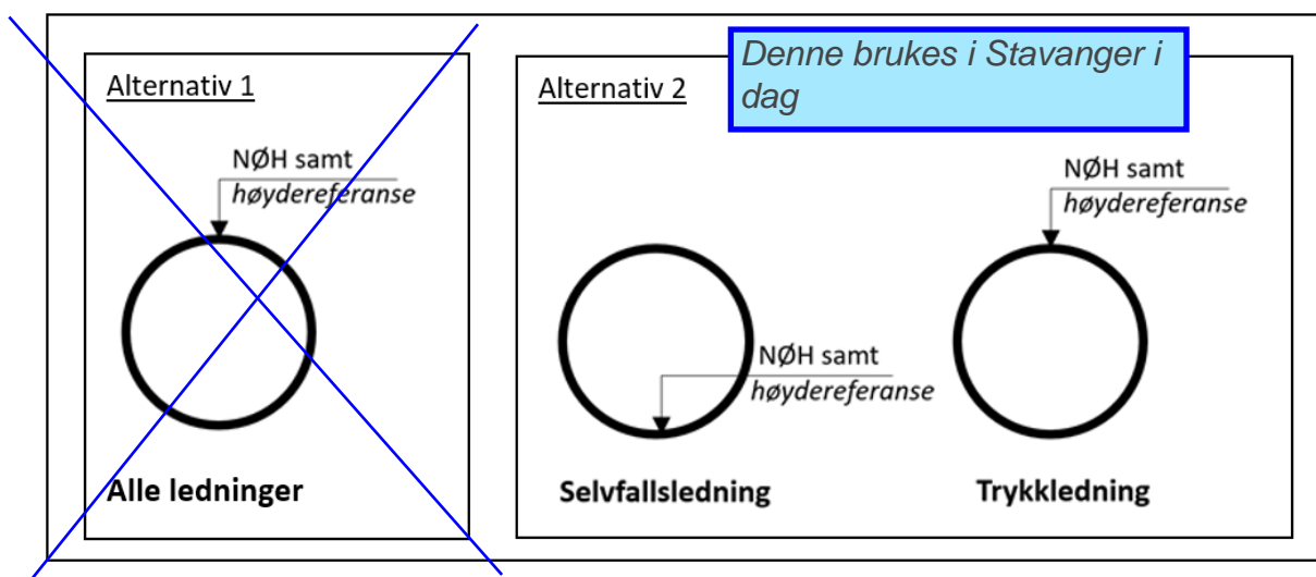
Figur 6. Hvordan måle inn ledning
